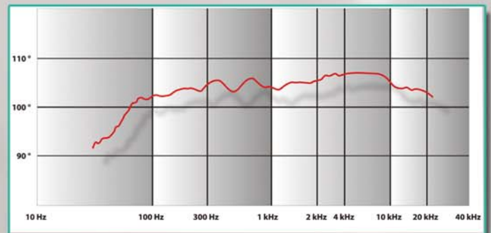
Frequenzgang der LA 210 ohne Audioprocessor.
